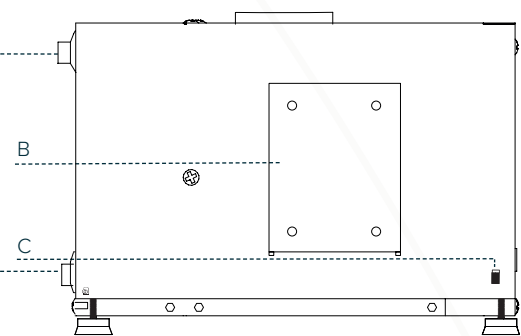
ACHTERAANZICHT
